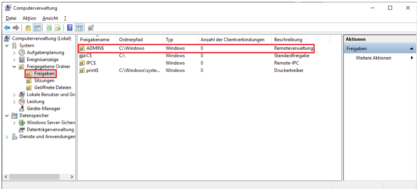
Abbildung 11 – Computerverwaltung - Freigabe
