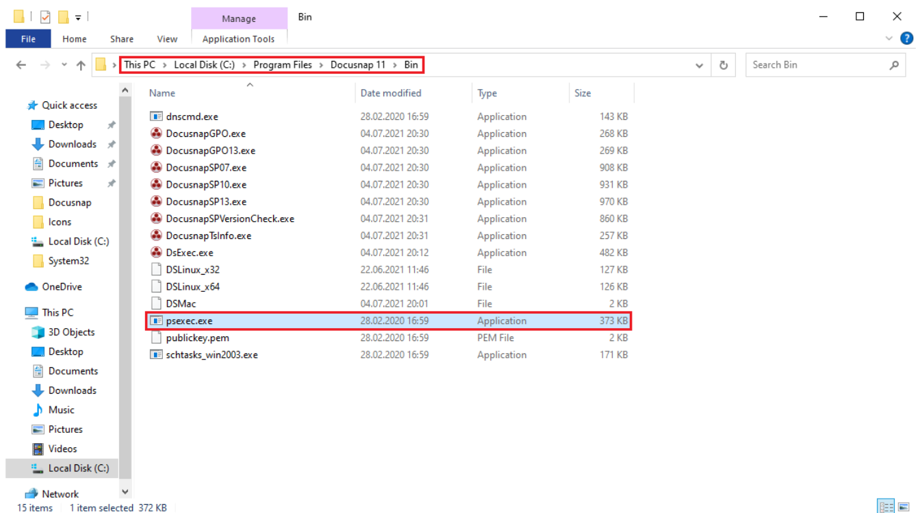
Abbildung 2 - PSEXec Pfad
