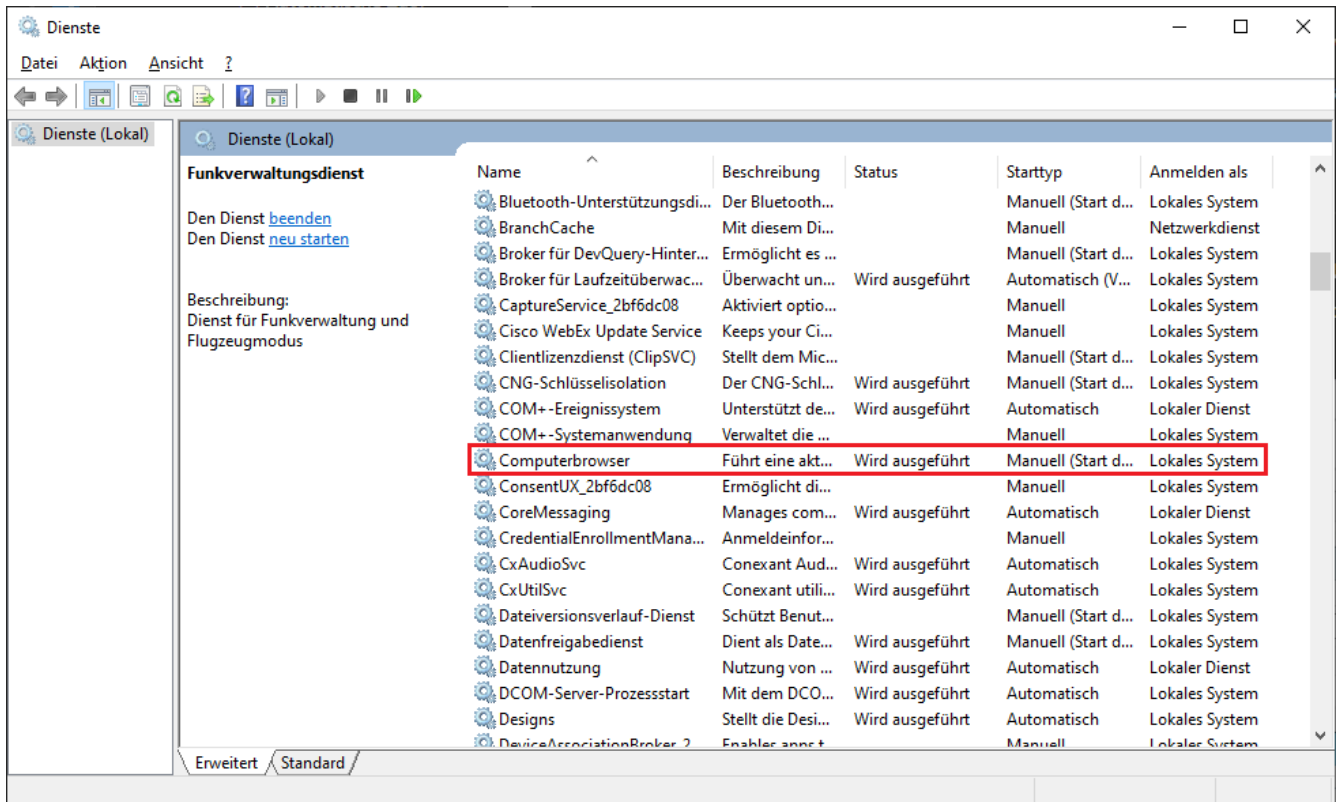
Abbildung 14 - Computerbrowser
