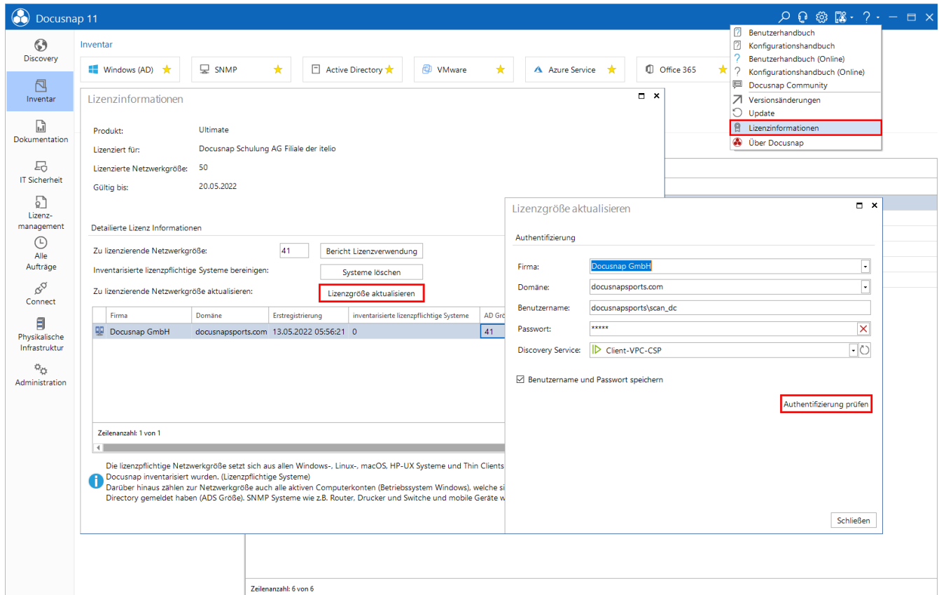
Abbildung 1 - Lizenzgröße aktualisieren
