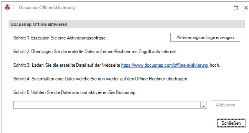
Abbildung 2: Offline Aktivierung
