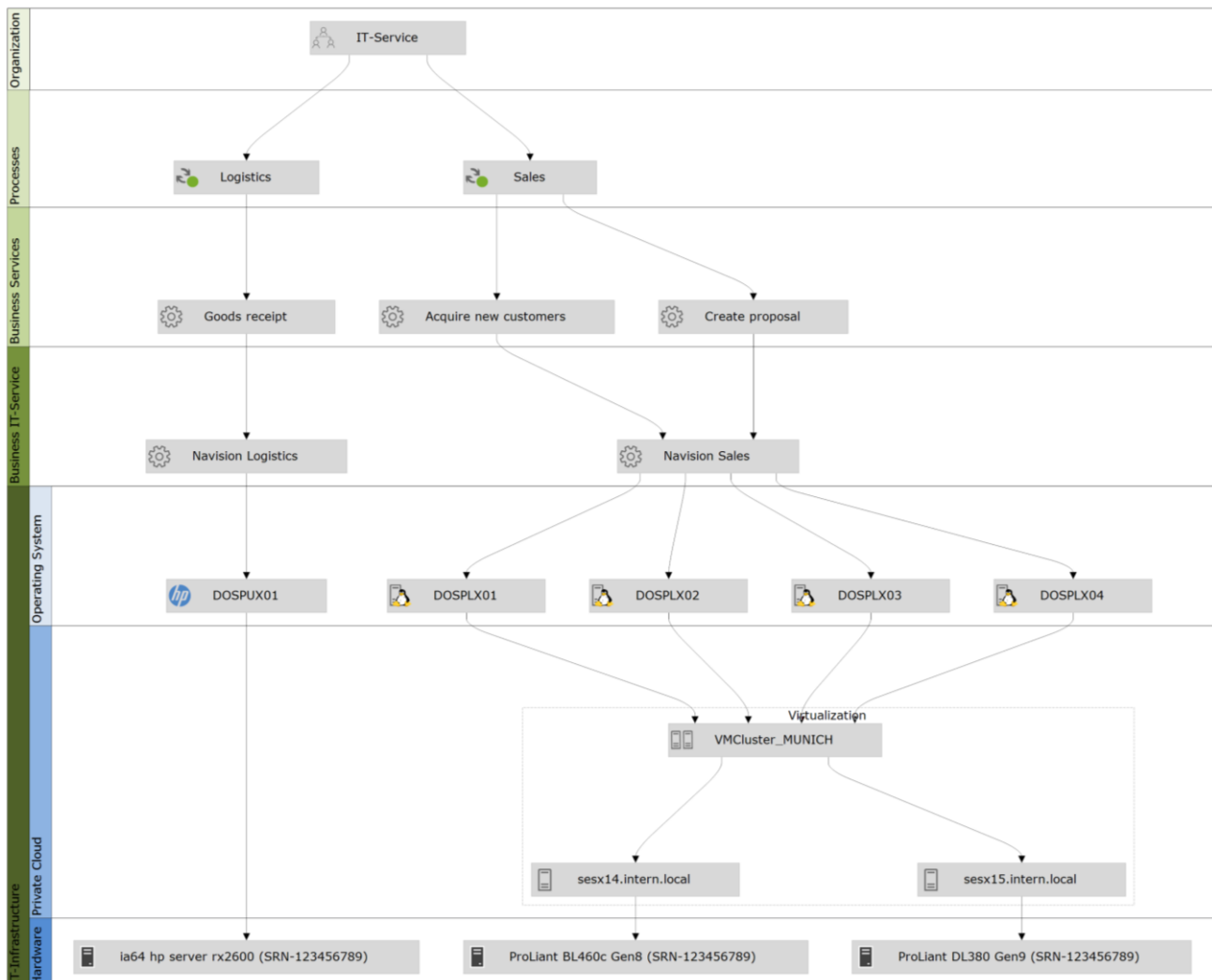
Abbildung 1 - Beispiel einer IT-Dokumentation
