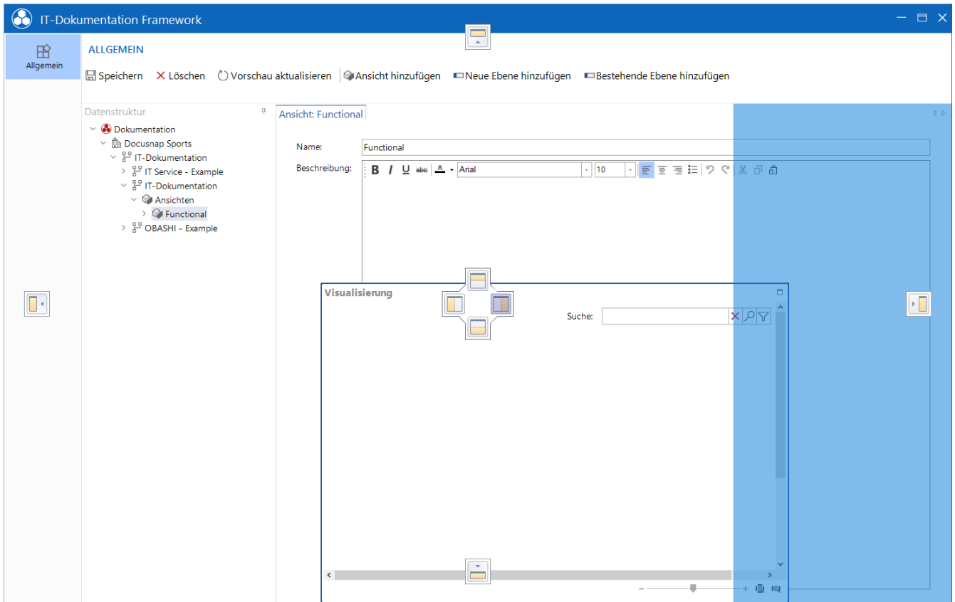
Abbildung 4 - Positionieren des Visualisierungs-Fensters
